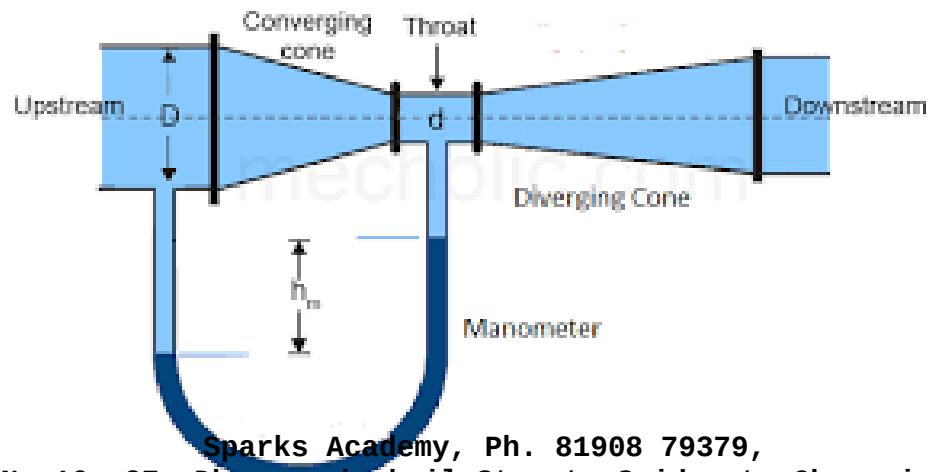
Venturimeter
