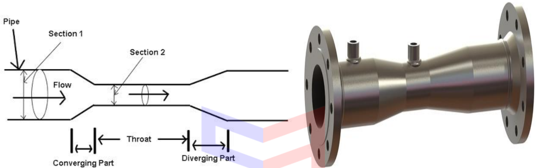
Venturimeter
